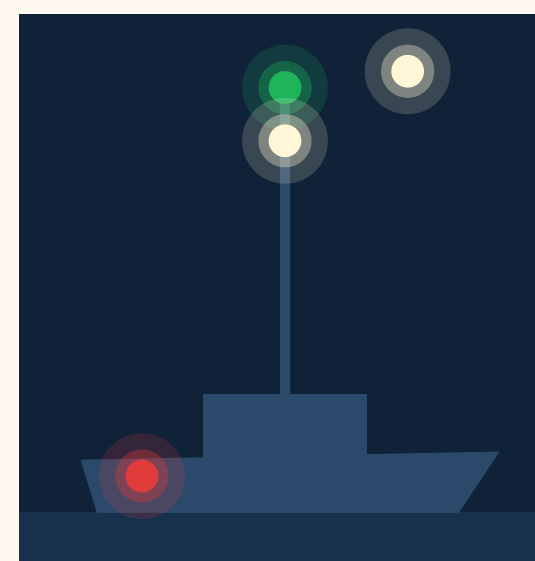
sinistro, oltre 50 m
