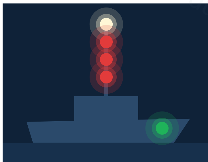
E · Condizionata dall'immersione, lato dritto
