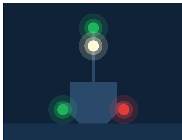
A · Pesca a strascico in abbrivio, di prora
