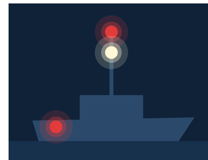
C · Pesca non a strascico, lato sinistro
