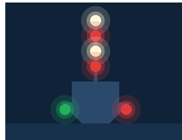
C · Manovrabilità limitata, di prora
