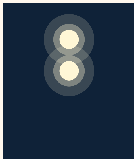
rimorchiatore: due testa d'albero in verticale
