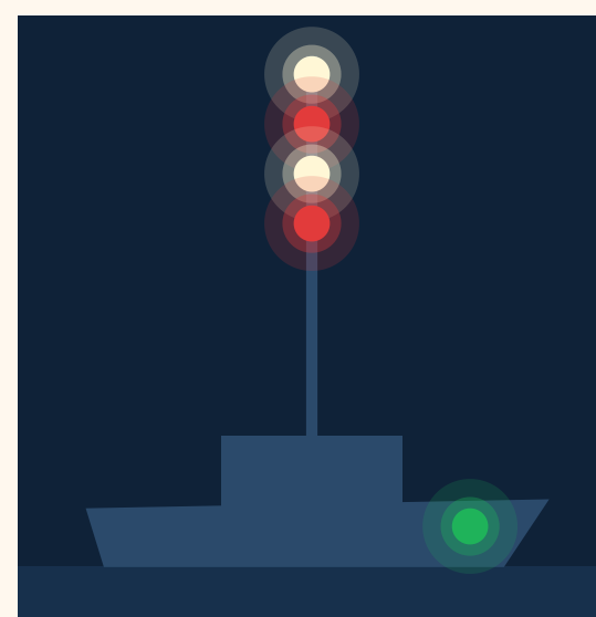
manovrabilità limitata, dritta
